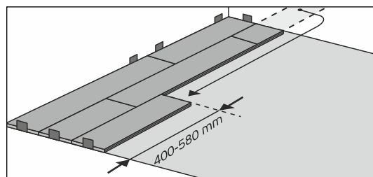
7.9 Каждый последующий ряд начинайте с части плашки, оставшейся от предыдущего ряда при выполнении условий п.7.7.
