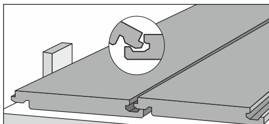
7.6 Первая плашка второго ряда вставляется в замок первого ряда по всей длине и защелкивается.
