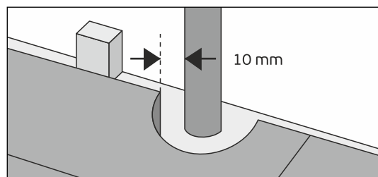
7.10 Возможно, придётся обрезать последний ряд - для более качественной укладки измеряйте ширину элемента с двух сторон, учитывая деформационный зазор 10 мм.
