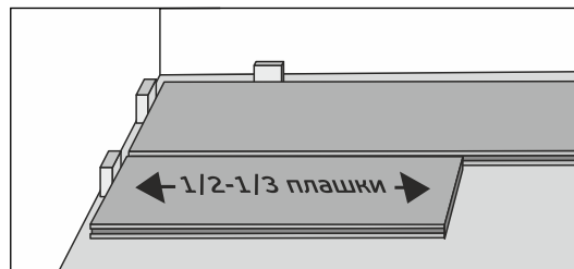
7.7 Рекомендуемое смещение плашек относительно соседних рядов — на 1/2 - 1/3 плашки.
