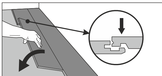
7.8 Аккуратно поместите плашку вплотную к короткому концу предыдущей плашки и защелкните замок одним движением. При необходимости воспользуйтесь резиновой киянкой.
